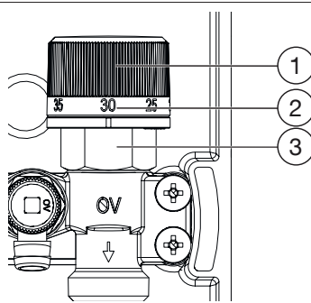
Abb. 4: Handrad
