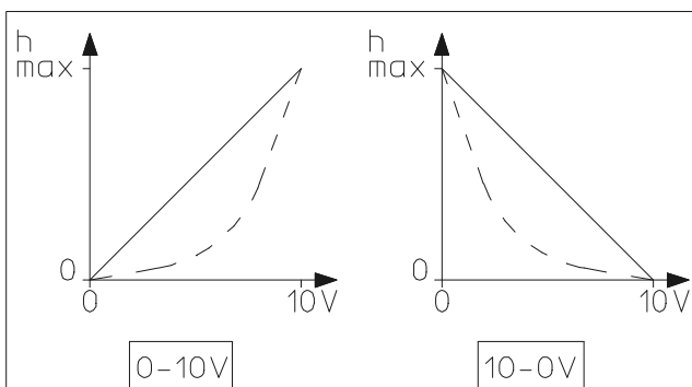
Abb. 5: Kennlinien Invertierung DIP-Schalter 7
