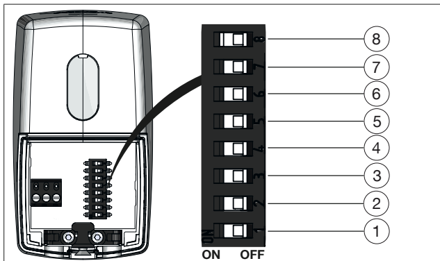
Abb. 4: DIP-Schalter
