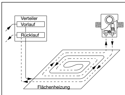
Einbauskeizze
