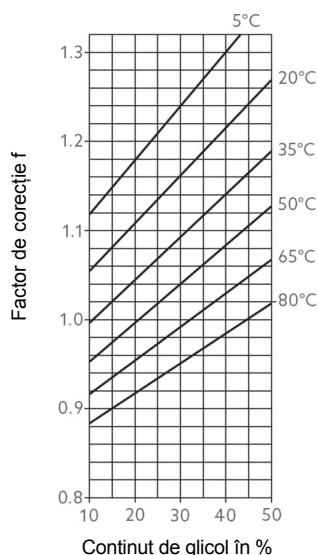
Factor de corecție f pentru etilenglicol
