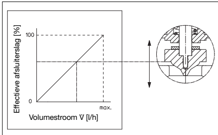
Afb. 5.3 Karakteristiek van de regelenheid 'Cocon QTZ'
