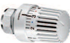
8 „Uni LR“, Cod. 161 63 01, (M 33 x 2,0), adatto per Rossweiner
