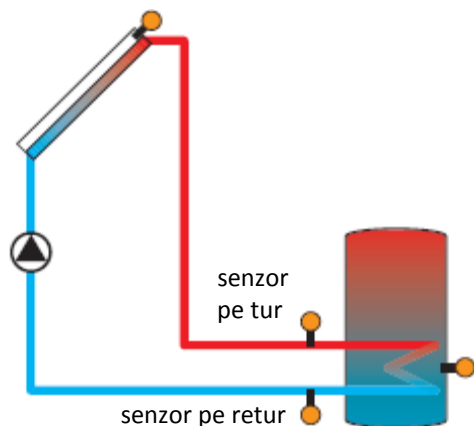
Exemplu de pozitionare a senzorilor pe tur și retur
