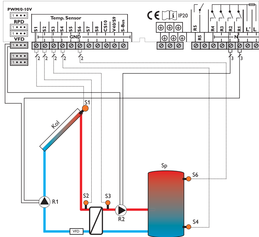
Beispiel für den elektrischen Anschluss einer Hocheffizienzpumpe
