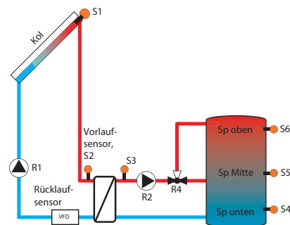
Beispiel für die Positionierung der Vor- und Rücklaufsensoren
