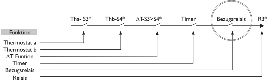
Bezugsrelais
