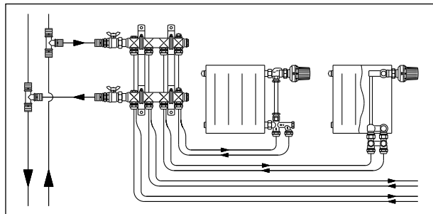
System-Darstellung Heizkörperanbindung
