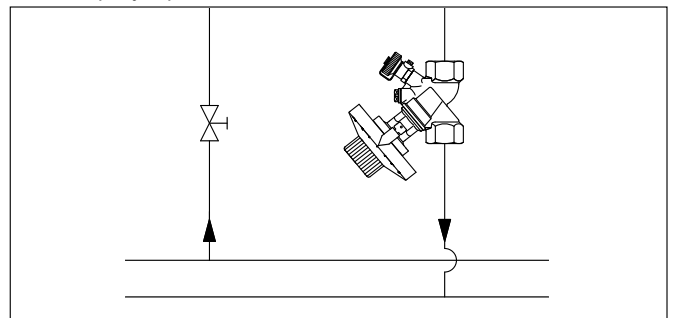
Пример: Регулирование расхода напр., в системе охлаждения. Преднастройка на регуляторе легко считывается.
