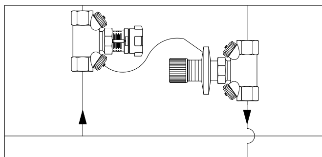
Пример: Регулирование перепада давления и ограничение расхода в системе без преднастроенных термостатических вентилей.
