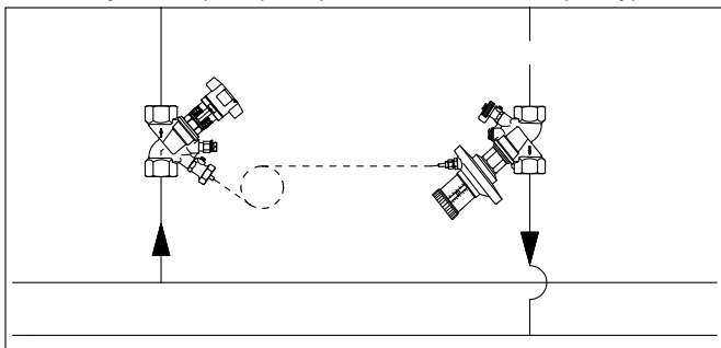
Пример: Регулирование перепада давления с ограничением расхода в системе без преднастраиваемых термостатических вентилей.
