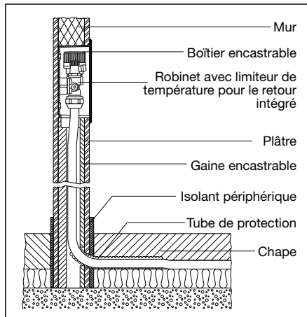
Coupe
