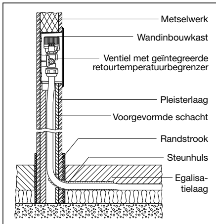
Doorsnede
