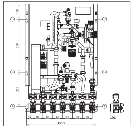
Abb. 5.1 Anschlussschema Kugelhahnanschlussleiste 1341080
