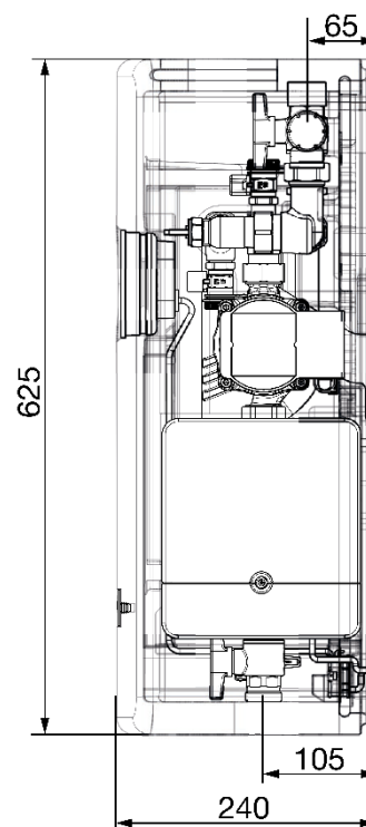
Afmetingen Regumaq X-45 (zijkant)
