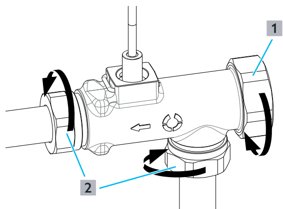
Fig. 22: Démontage du capteur de débit
