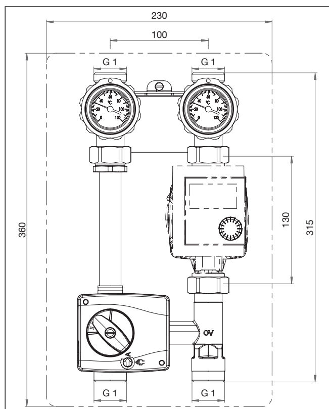
Dimensioni „Regumat M3-130“ DN 20
