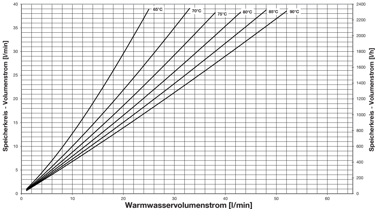
Abb. 47: Volumenstrom Speicherkreis - Trinkwassererwärmung auf 65 °C
