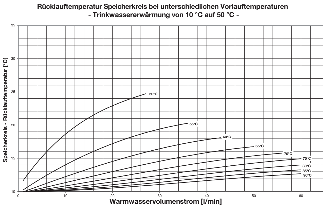
Abb. 42: Rücklauftemperatur Speicherkreis - Trinkwassererwärmung auf 50 °C
