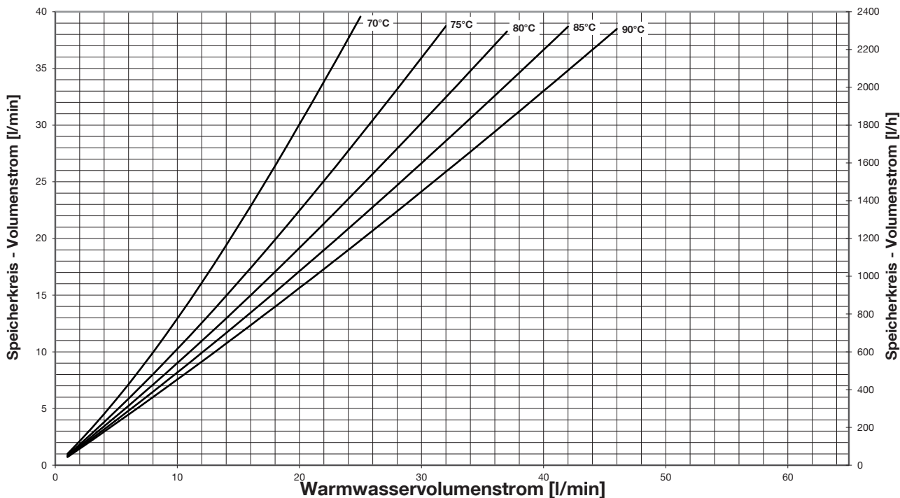
Abb. 49: Volumenstrom Speicherkreis - Trinkwassererwärmung auf 70 °C
