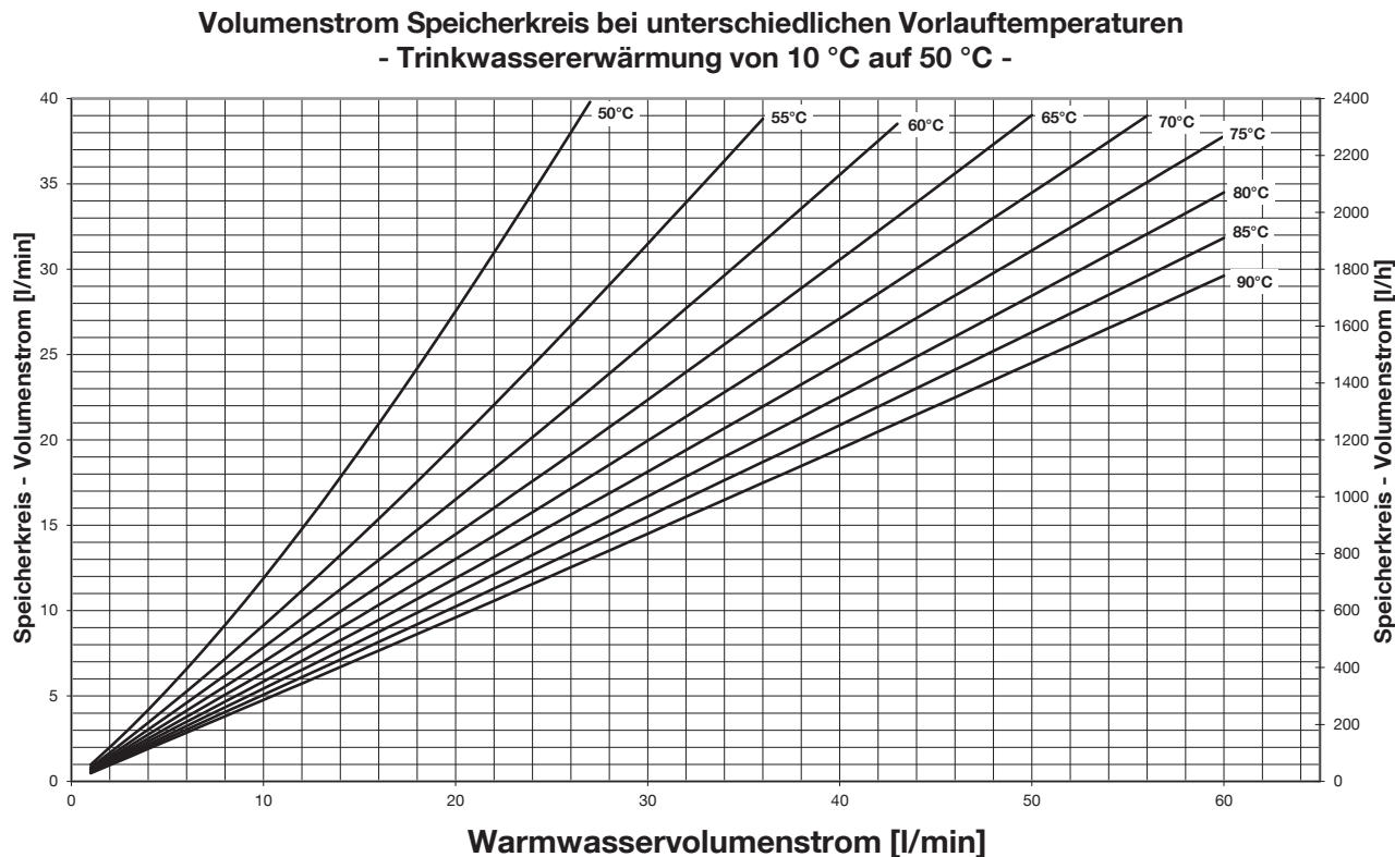
Abb. 41: Volumenstrom Speicherkreis - Trinkwassererwärmung auf 50 °C
