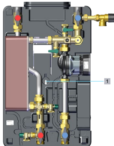
Fig. 13: Position de la rondelle
