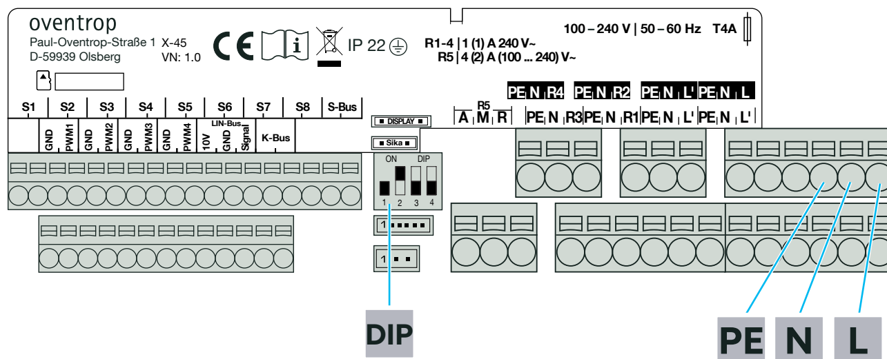
Fig. 9: Affectation des bornes
