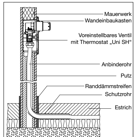
Abb. 5.1 Schnitt „Unibox T SH“ in Wand
