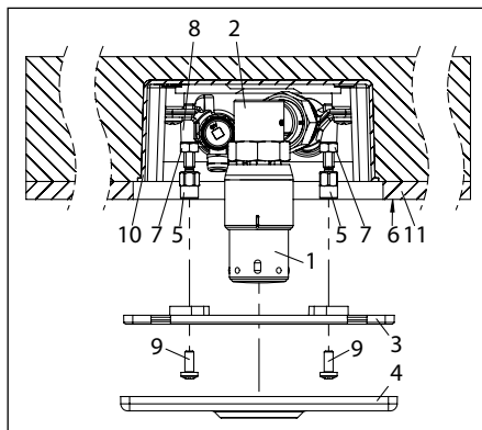
Afb. 5.4 Uitleinen van de stelpennen
