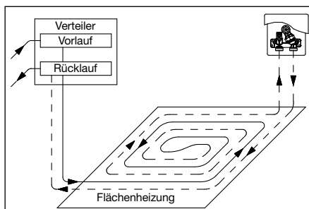
Abb. 5.3 Einbauskizze
