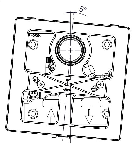
Afb. 5.6 Hoekverstelling
