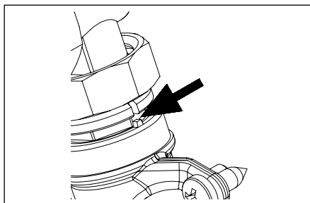
Abb. 6.3 Ausrichtung des Winkeladapters
