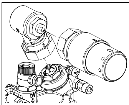
Abb. 6.1 Winkeladapter auf Ventilgehäuse
