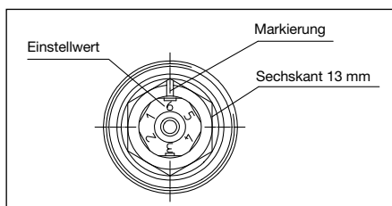
Abb. 6.2 Voreinstellbarer Ventileinsatz
