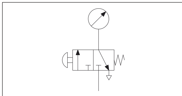
Schema de conectare
