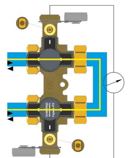
Измерване на диференциалното налягане, напр. с OV-DMC 3
