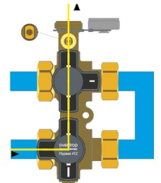
Източване от страна на инсталацията/уреда, обезвъздушаване и промиване от страна на инсталацията
