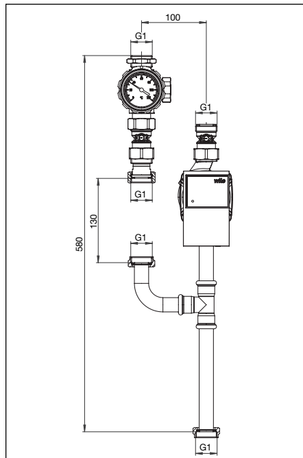
Fig. 4.3 Encombrements
