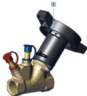
Fig. 3 - Posizione clip limitatrice
