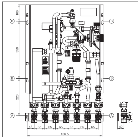
Abb. 5.1 Anschlusschema Kugelhahnanschlussleiste 1341080
