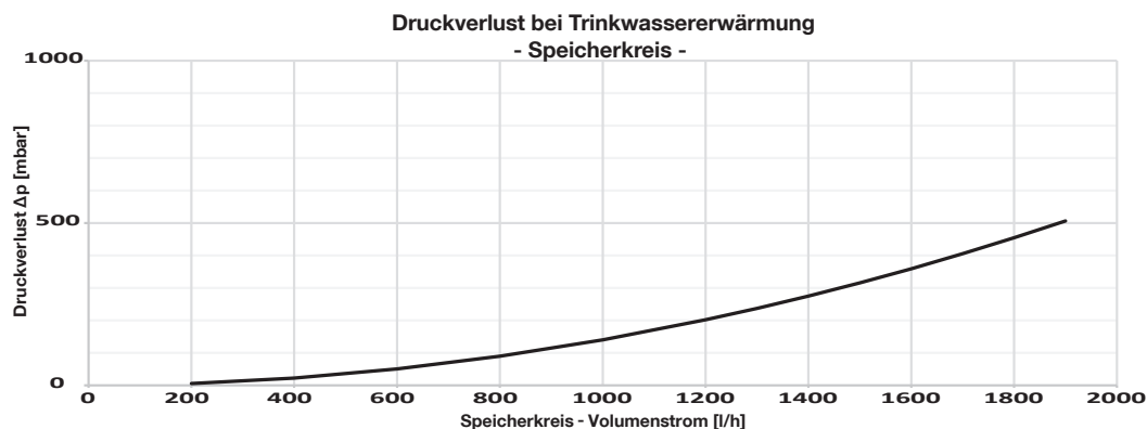
Abb. 40: Kennlinie Druckverlust bei Trinkwassererwärmung (Speicherkreis)
