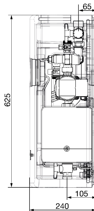
Abmessungen Regumaq X-45 (Seite)
