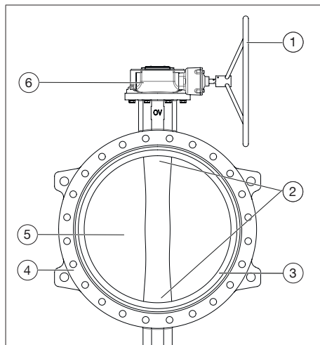
Fig. 2: Construction vanne papillon (modèle à double bride) à réducteur à volant DN 700 - DN 1400
