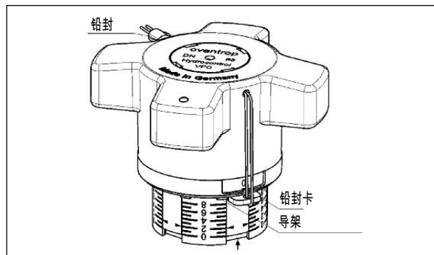
图 7.2 手轮的锁定
