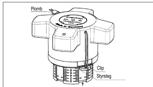
Bild 7.2 Blockering av handhjulet
