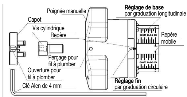
Fig. 7.1 Pré-réglage
