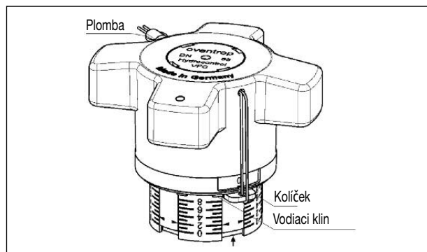
Obr. 7.2 Blokovanie ručného koleska
