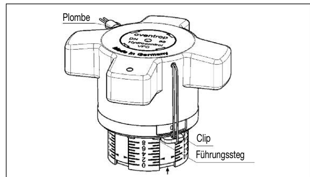
Abb. 7.2 Blockierung des Handrades
