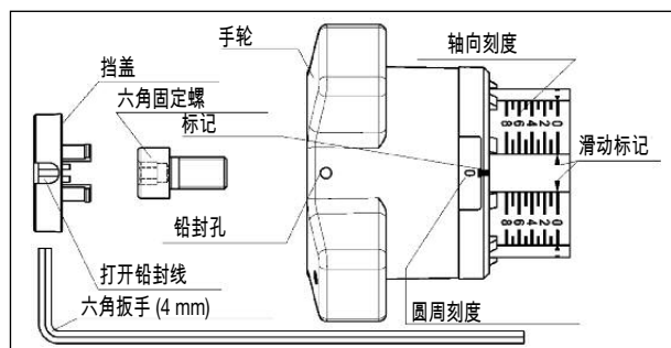
图 7.1 预设
