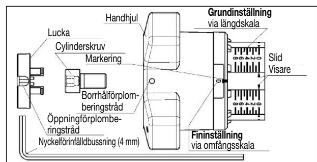
Bild 7.1 Förinställning
