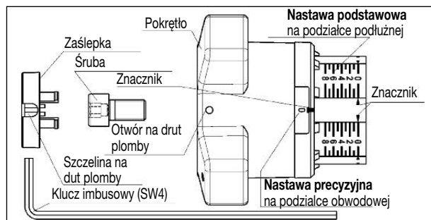
Rys. 7.1 Nastawa wstępna
