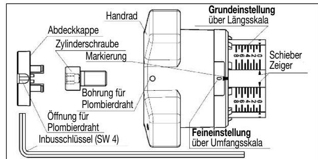
Abb. 7.1 Voreinstellung
