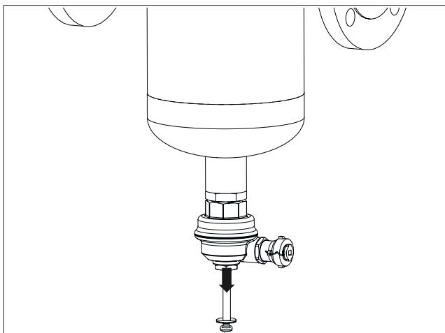
Fig. 4: Magnet
