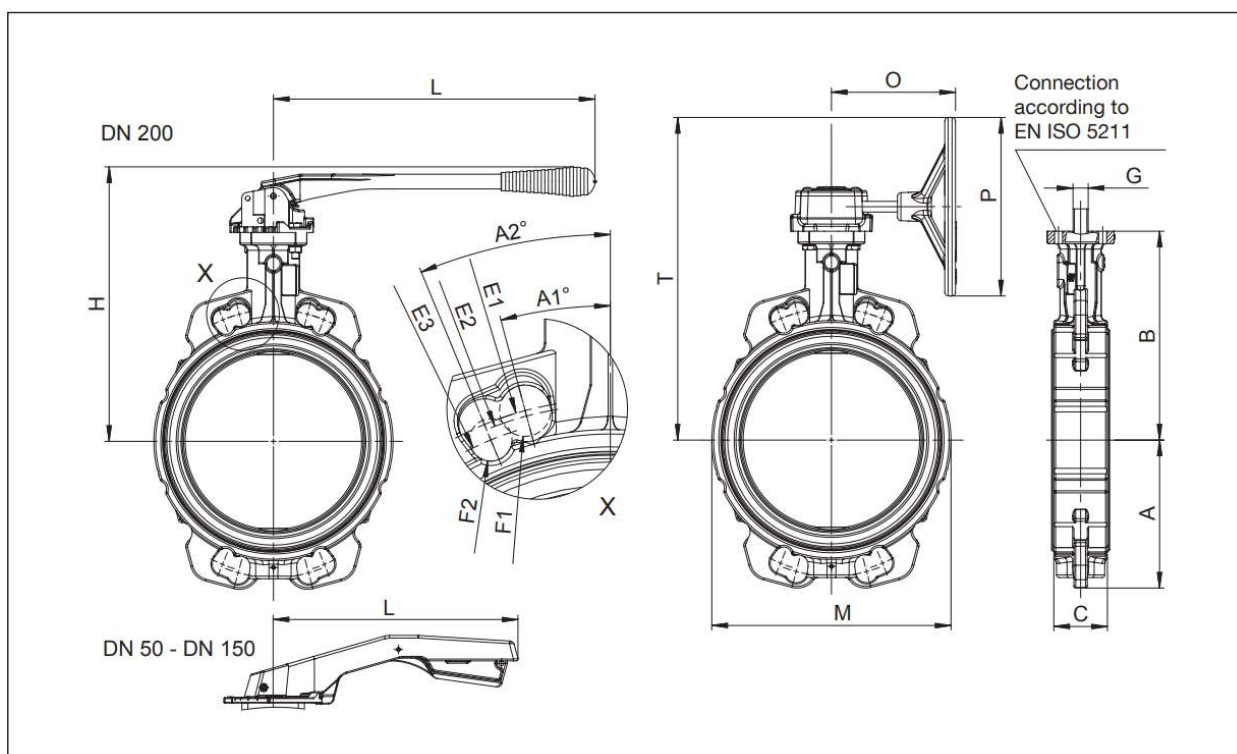
Uzavírací středová klapka (DN 50 až DN 300)
