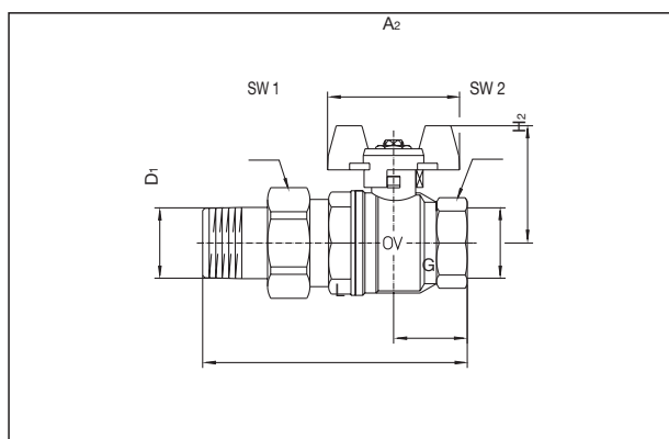
Méretetek, cikkszám: 1075804-10 (DN 15 - DN 32) fém pillangó fogantyú (max. DN 25 Al, DN 32 horganyzott acél)
