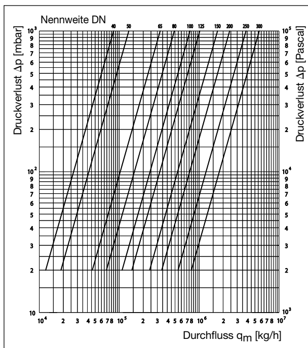
Durchflussdiagramm
