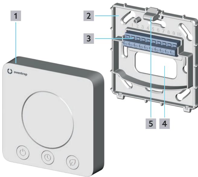
Abb. 3: Aufbau
