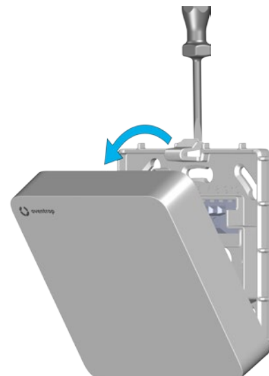
Abb. 5: Montageplatte lösen
