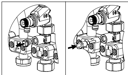
Fig. 6.2 Montaggio sonda per contacalorie
