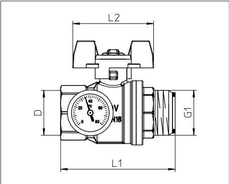
Fig. 5: Dimensions robinet à tournant sphérique
