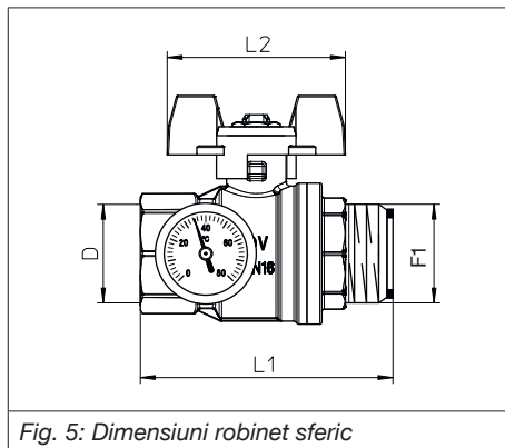
Fig. 5: Dimensiuni robinet sferic
