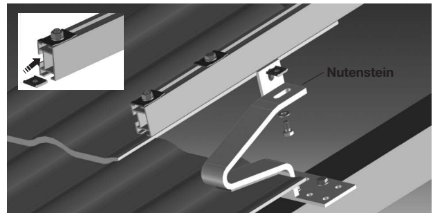
Abb. 7: Montageschienen montieren
