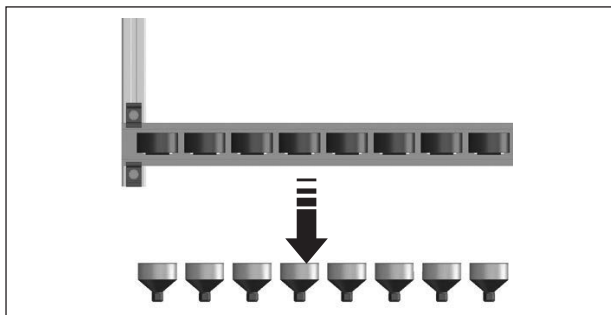
Abb. 18: Kunststoffkappen aus den Röhrenhaltern schrauben
