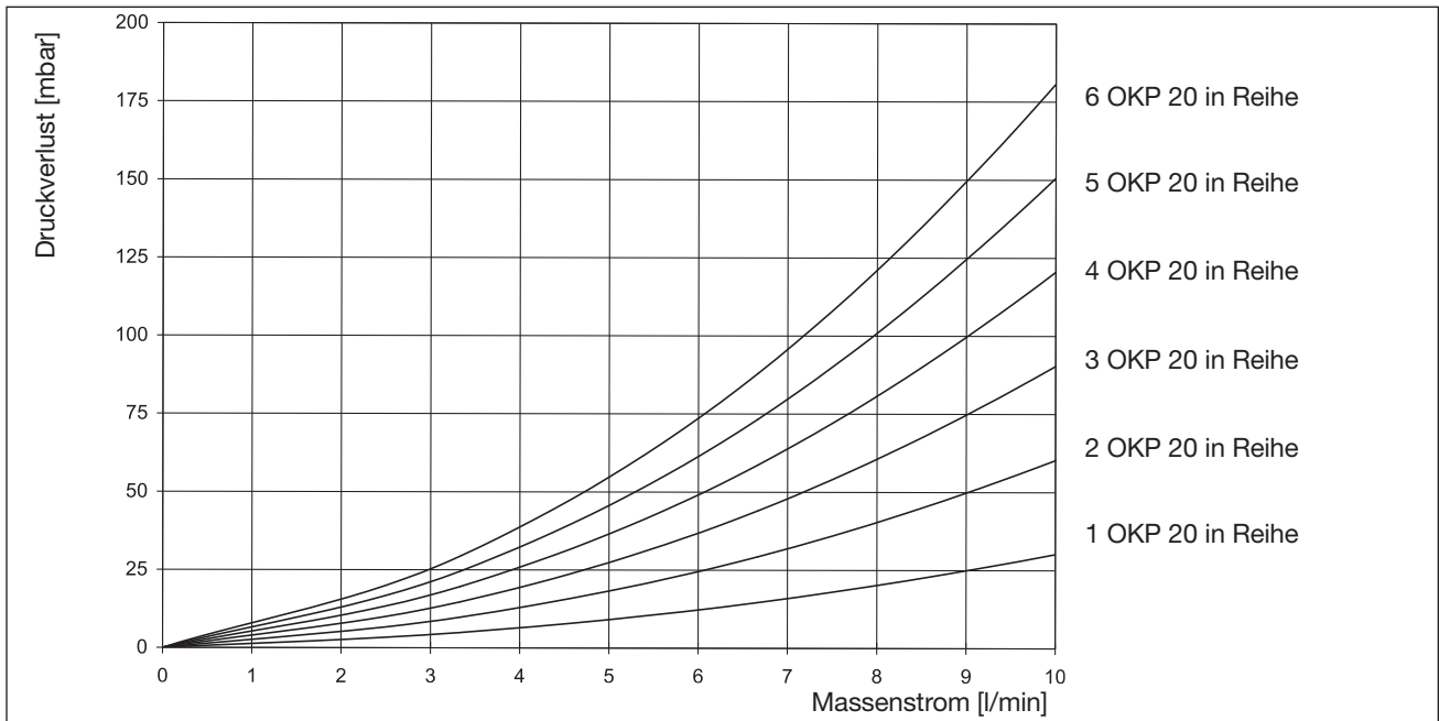
Diagramm 1: Druckverluste Wärmeträgerflüssigkeit „Tyfocor LS“ bei 40°C Druckverlustangaben ohne Verbindungs- und Anschlussschläuche
