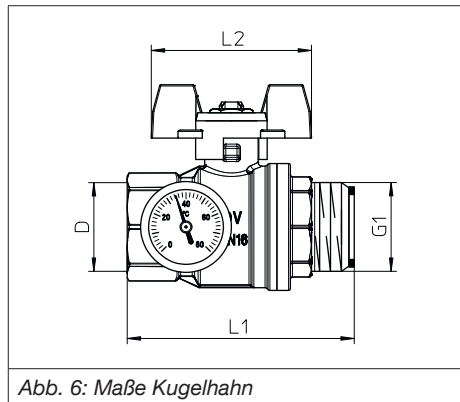
Abb. 6: Maße Kugelhahn
