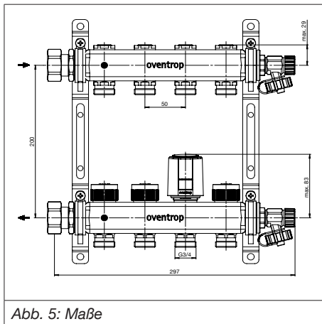
Abb. 5: Maße
