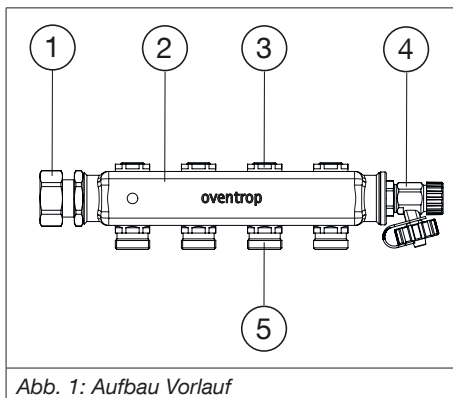
Abb. 1: Aufbau Vorlauf
