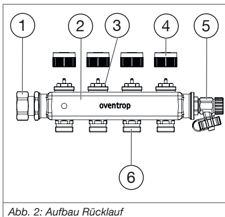
Abb. 2: Aufbau Rücklauf
