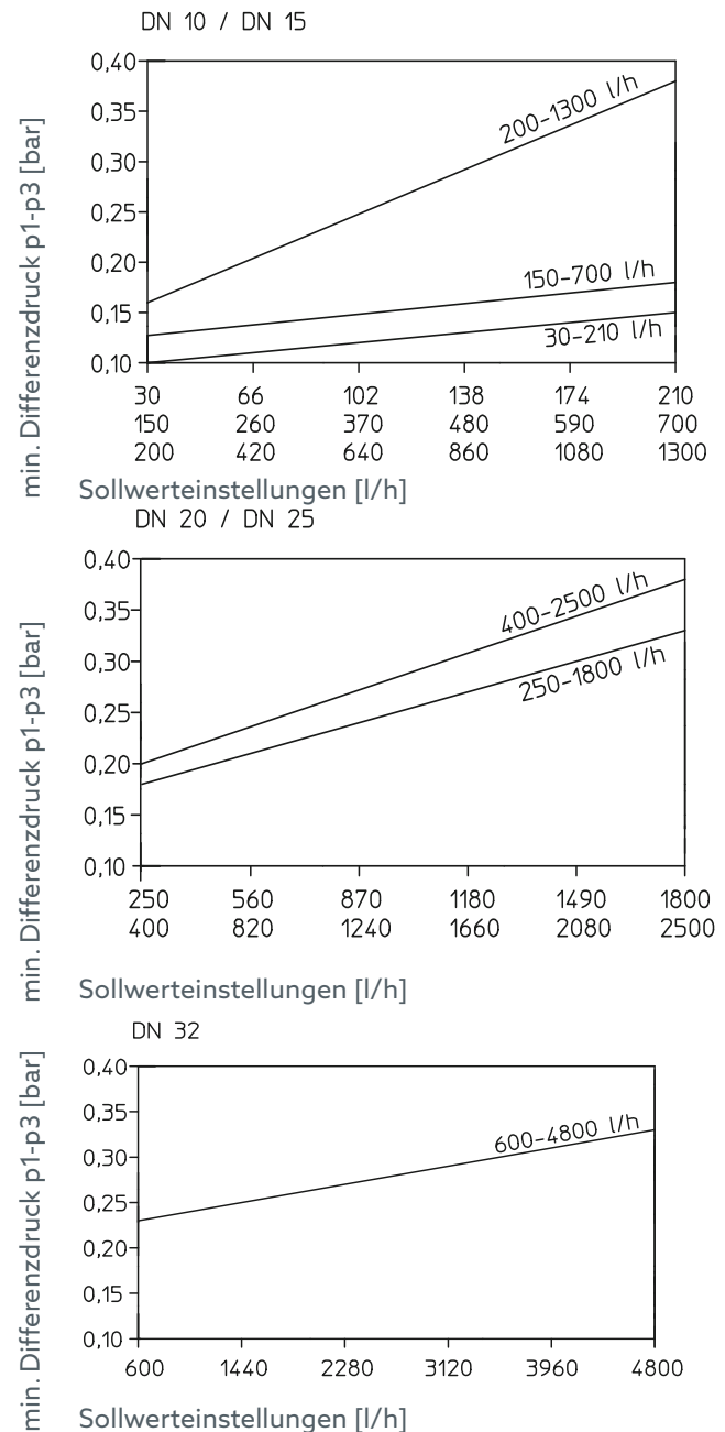
Abb. 13: Mindest-Differenzdrücke
