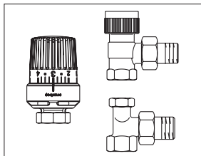
Obr. 1 Termostatický ventil-sada, rohové provedení
