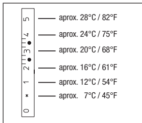
Fig. 5 Escala de temperatura del termostato "Uni LH"
