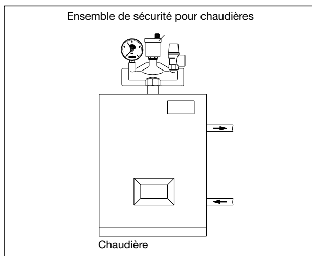
Schéma d'installation
