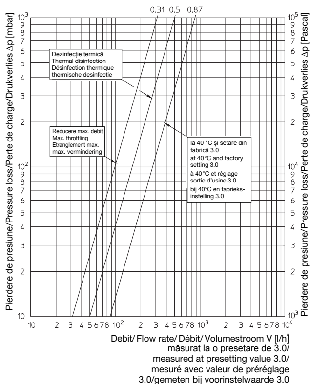
„Aquaström T plus” DN 20
