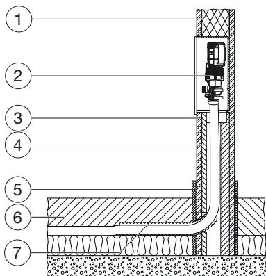
Abb. 8: Einbauquerschnitt
