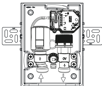
Abb. 10: „Unibox TQ-RTL R-Tronic“ mit Winkeln
