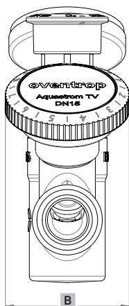
Рис. 3: Размеры спереди
