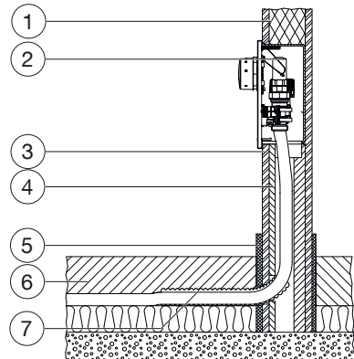
Abb. 8: Einbauquerschnitt
