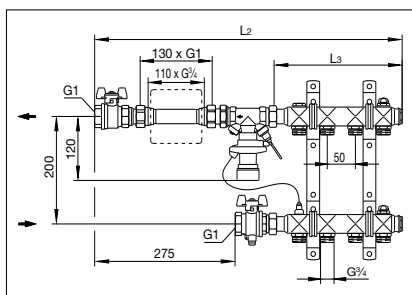
Fig. 5: Set di collegamento contacalorie Set 2, dritto e collettore inox „Multidis SH“ per collegamento radiatori, lunghezze d'installazione
