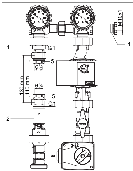
Fig. 5.2 Encombrements du jeu de montage pour compteurs de calories
