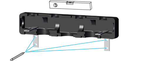
Abb. 5: Bohrlöcher markieren
