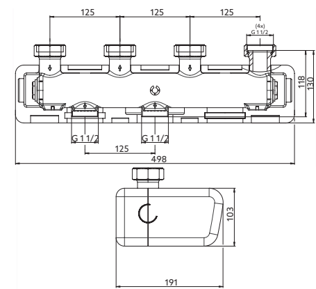
Fig. 2: Encombrements
