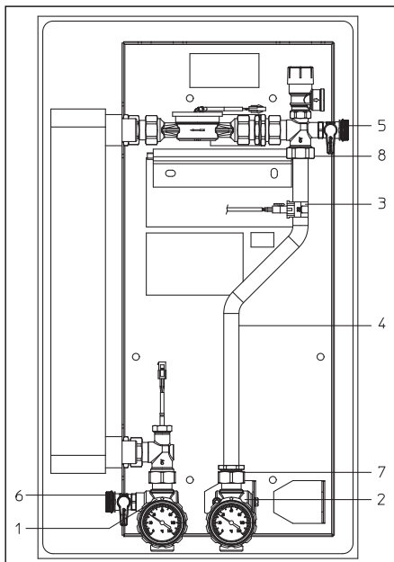
Abb. 1: Frischwasserstation „Regumaq X 30“ im Auslieferungszustand (Darstellung Sekundärkreis)
