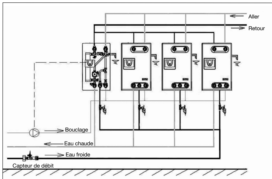
Illustr. 3 : Exemple d'installation – Commande de cascade se composant de:
