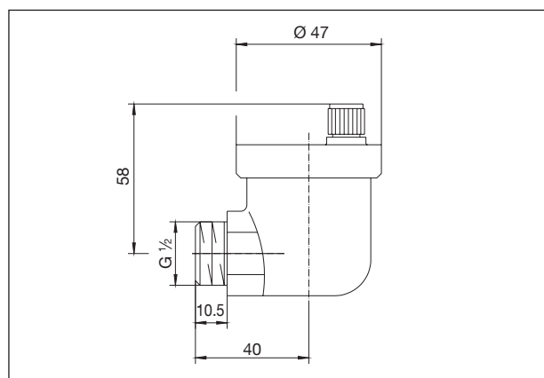
Encombrements réf. 1088404
