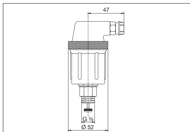
Encombrements réf. 1088203
