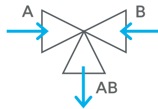
Toepassing als mengafsluiter: stromen A en B worden naar AB gemengd, afhankelijk van de stand
